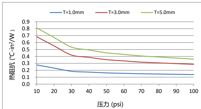
热阻抗
