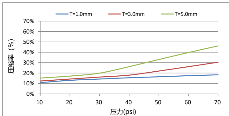
压缩率
