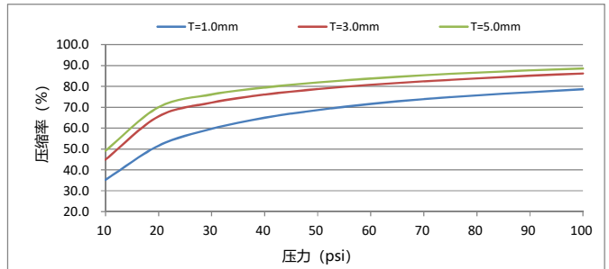
压缩率
