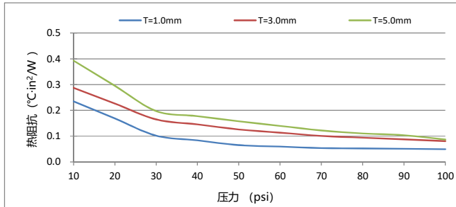
热阻抗
