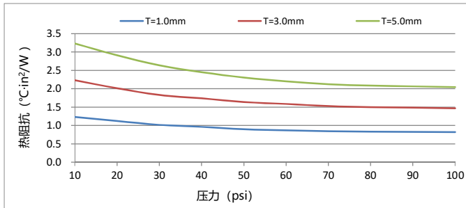
热阻抗
