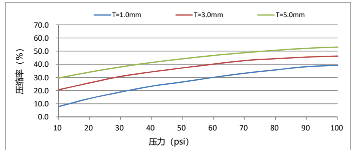
压缩率
