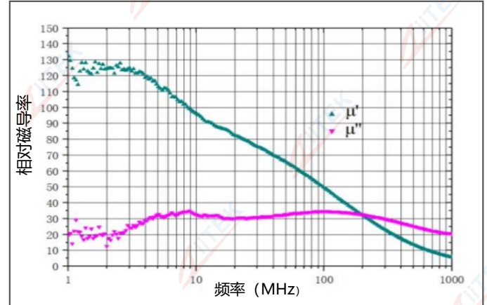
材料磁谱
