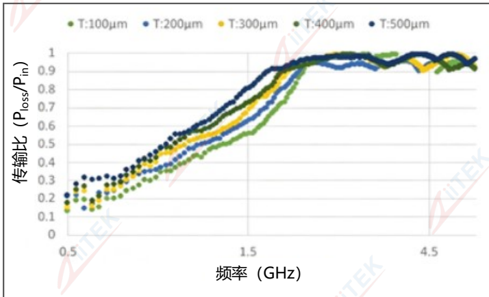
衰减特性
